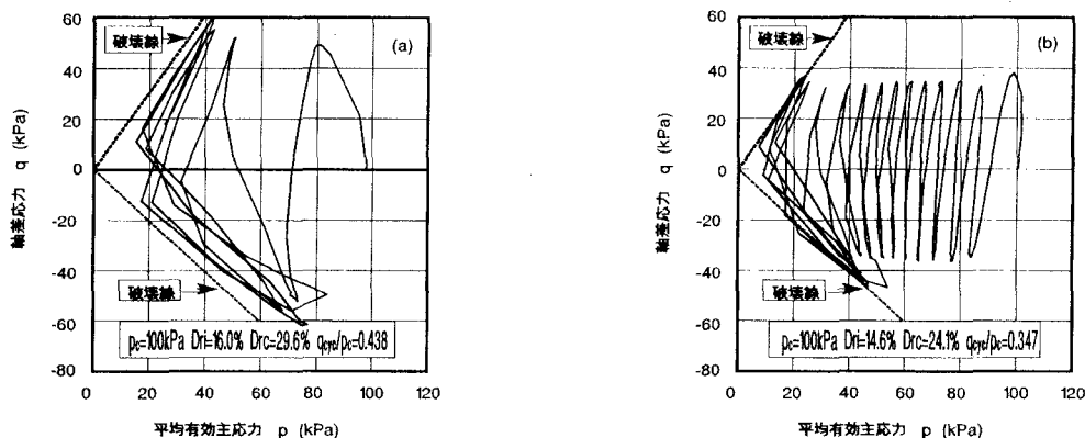
図-3 繰返し有効応力経路
