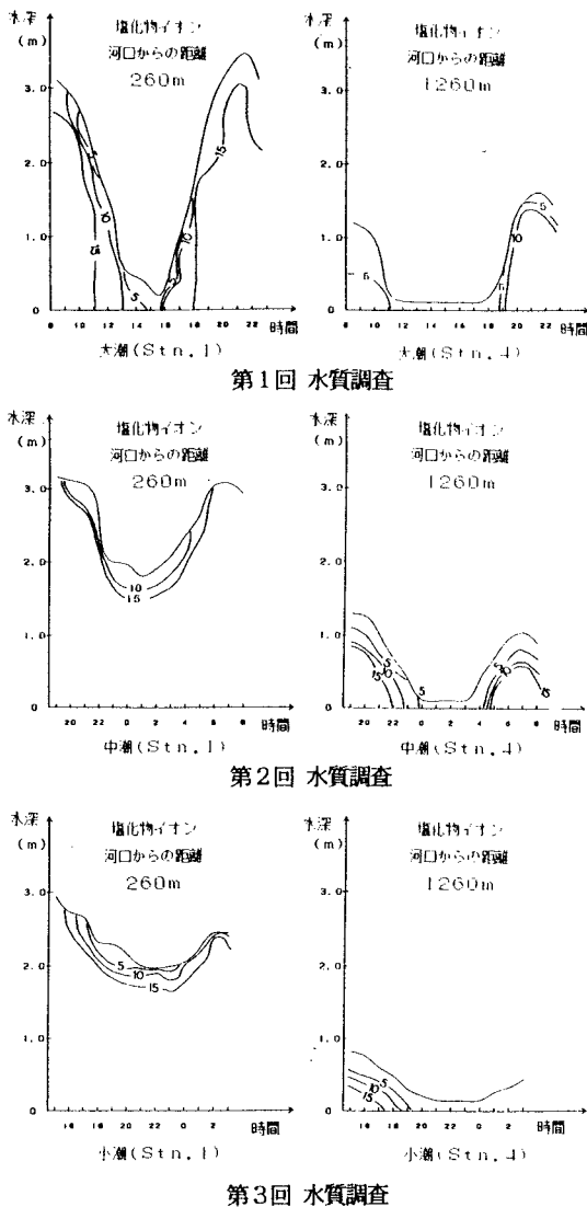
図1 塩化物イオン横断面図
