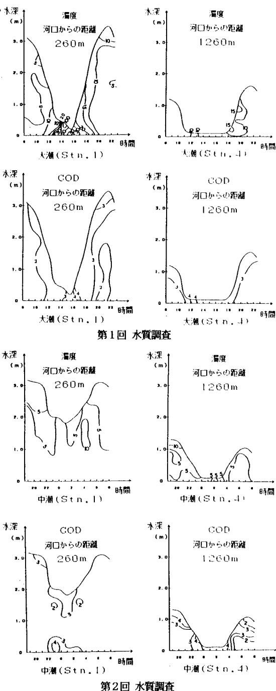
第2回 水質調査 図2 濁度、COD横断面図
