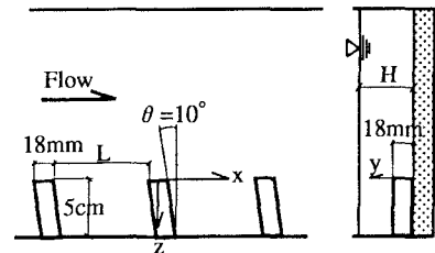
図-1 水制概要
