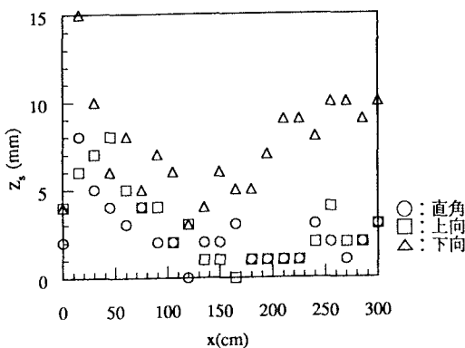
図-2 極大洗掘深 z_s の流下方向変化
