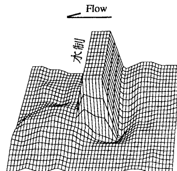
図-3 直角水制周辺の鳥瞰図
