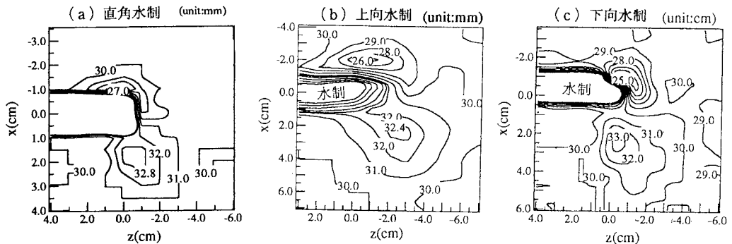
図-4 河床高の等値線
