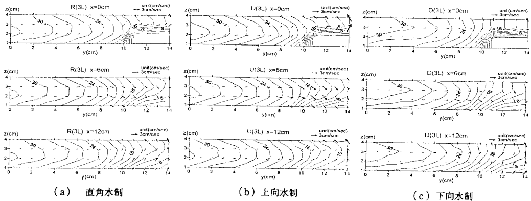
図-5 主流速の等値線および二次流ベクトル
