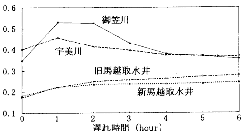
図－5 降雨との相関関数
