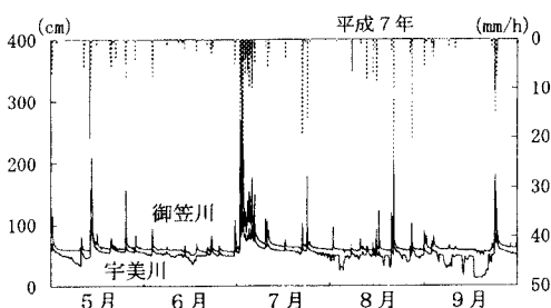
図－3 河川の水深変動
