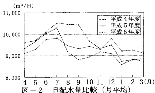
図－2 日配水量比較（月平均）
