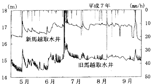
図－4 取水井の水位変動
