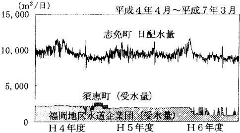
図－1 日配水量時系列
