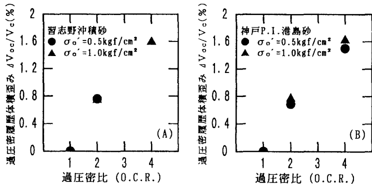
図-4 過圧密履歴体積歪み～過圧密比関係
