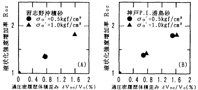
図-5 液状化強度増加率～過圧密履歴体積歪み関係
