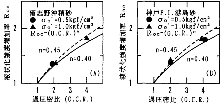
図-3 液状化強度増加率～過圧密比関係
