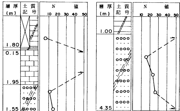
図-1 土質柱状図
