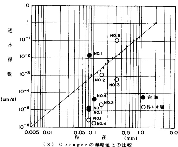
図-4 粒度と透水係数の関係
