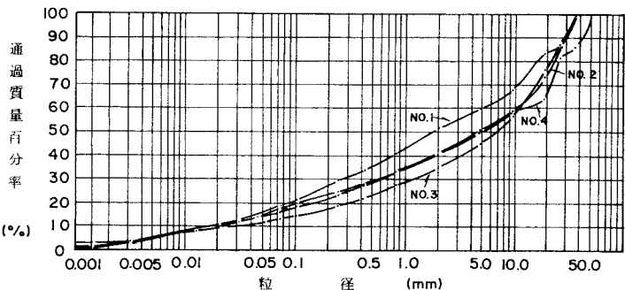
図-3 粒径加積曲線
