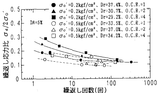
図-1(B) 繰返し回数～繰返し応力比関係
