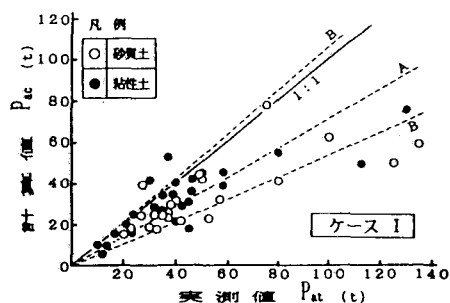
図-1 許容支持力の実測値と計算値の関係
