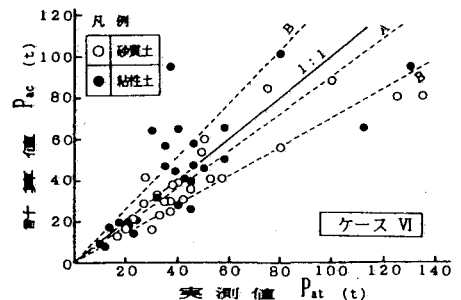
図-6 許容支持力の実測値と計算値の関係
