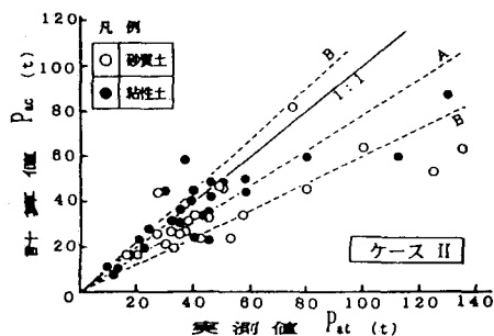
図-2 許容支持力の実測値と計算値の関係
