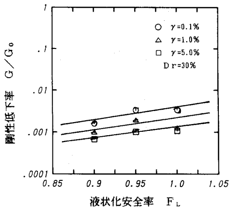
図-4 液状化安全率～剛性低下率の関係
