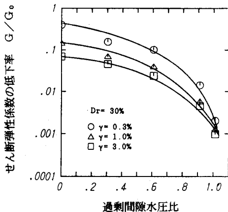
図-3 過剰間隙水圧比～せん断弾性係数の低下率の関係
