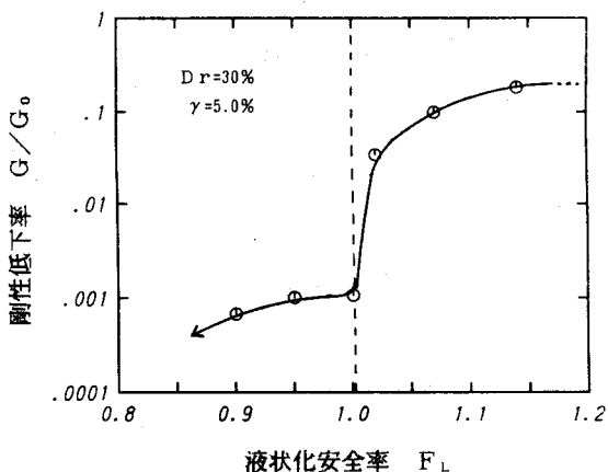
図-5 液状化の進行に伴う剛性低下
