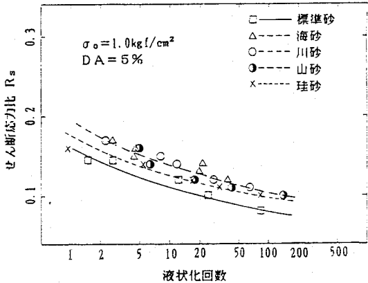
図-1 液状化強度曲線
