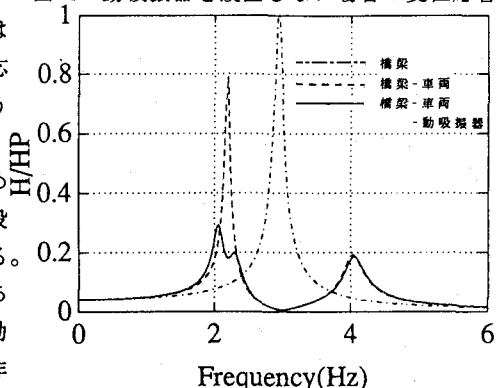
図-4 支間中心における周波数伝達関数
