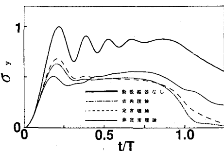
図-5(a) 非連成の場合の変位応答
