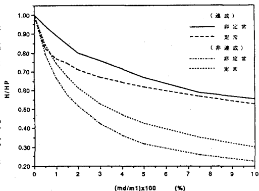
図-6 質量比による最大応答の変化
