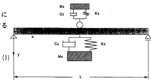
図-1 橋梁-車両-動吸振器
