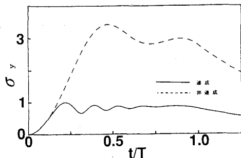
図-3 動吸振器を設置しない場合の変位応答
