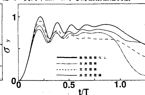
図-5(b) 連成の場合の変位応答
