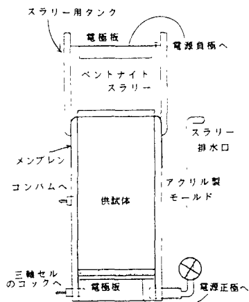
図-1 電気泳動装置
