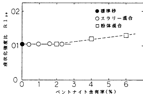
図-4 液状化強度比～ベントナイト含有率
