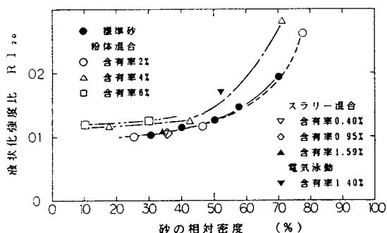
図-3 液状化強度比～相対密度
