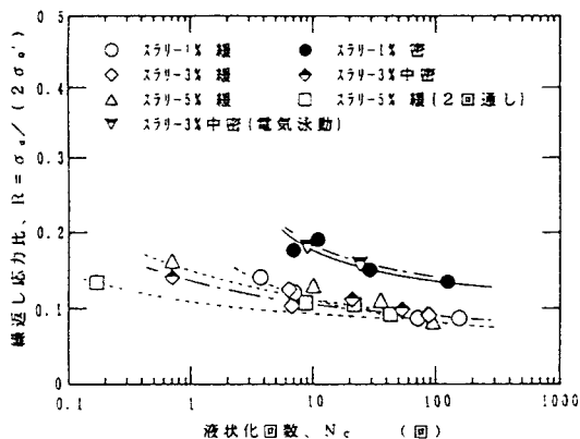
図-2(b) 応力比～液状化回数関係
