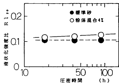
図-5 液状化強度比～圧密時間
