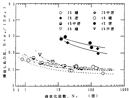
図-2(a) 応力比～液状化回数関係
