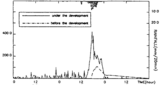
図-5 流域の開発による流出形態の変化の推定
