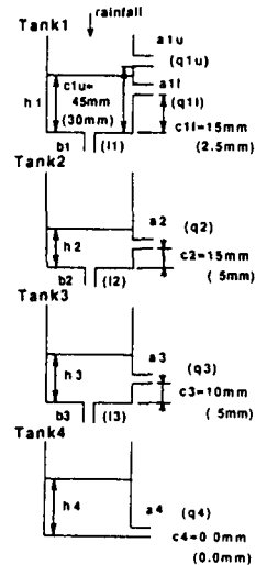
図-2 タンクモデル
