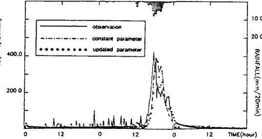
図-3(b) 開発中の流出解析例(CASE6)
