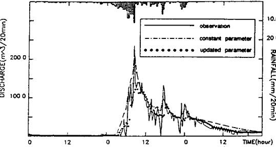
図-3(a) 開発前の流出解析例(CASE4)
