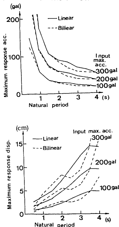
図2. バイリニア系と線形系の応答最大値の比較
