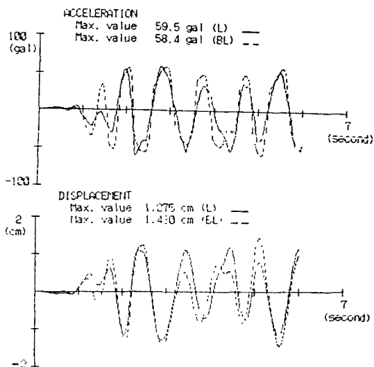
図1. バイリニア系と線形系の応答時刻歴の比較
