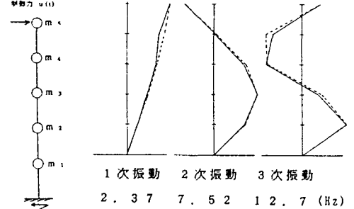
図-2 構造物モデルの振動モードと固有振動数
