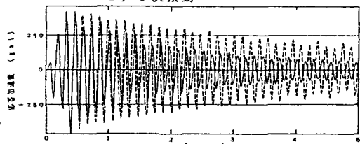
b) 2次振動
