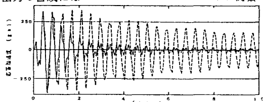
a) 1次振動
