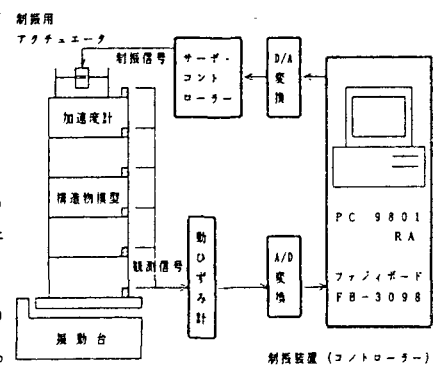
図-3 振動制御システム
