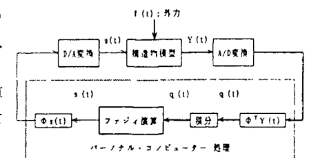
図-4 ファジィ・ボードを用いた制振システム
