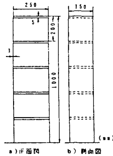
図-1 構造物モデルと制御モデル
