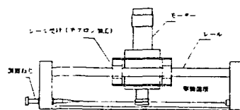
図-5 アクチュエータの概形
