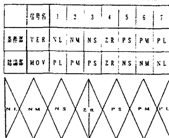
図-6 ファジィ演算のルールとメンバーシップ関数
