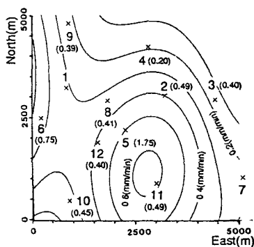
図-4 11時56分における1分先予測降雨分布
