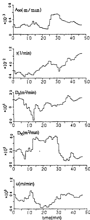
図-2 物理パラメーターの同定結果
