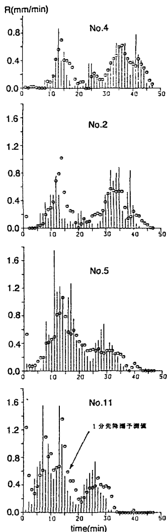
図-3 実測降雨時系列および1分先降雨予測値
