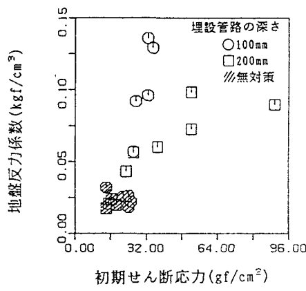
図3 地盤反力係数とせん断応力との関係
