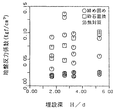
図4 地盤反力係数と埋設深さとの関係
