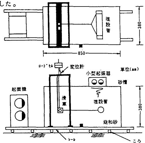
図1 振動砂槽と引き抜き試験装置
