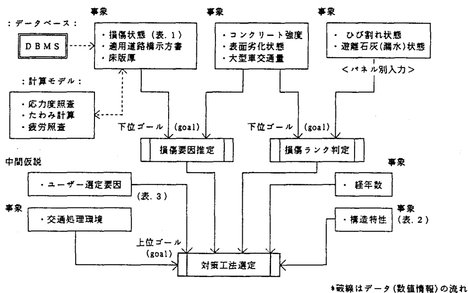
図. 2 エキスパートシステムのフロー
