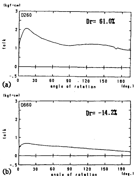
図-2 回転角-トルクの関係
