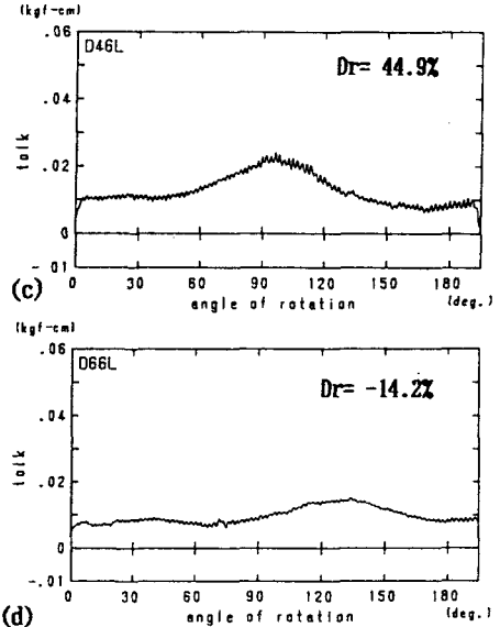
図-2 回転角-トルクの関係
