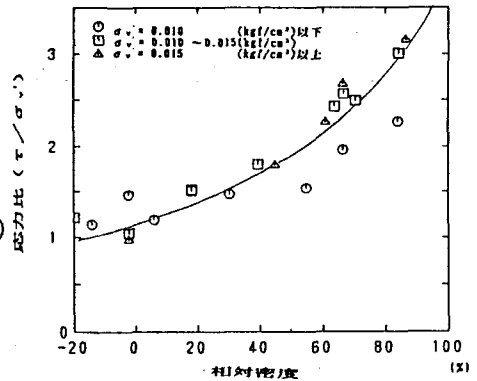
図-3 地盤密度とせん断強度
