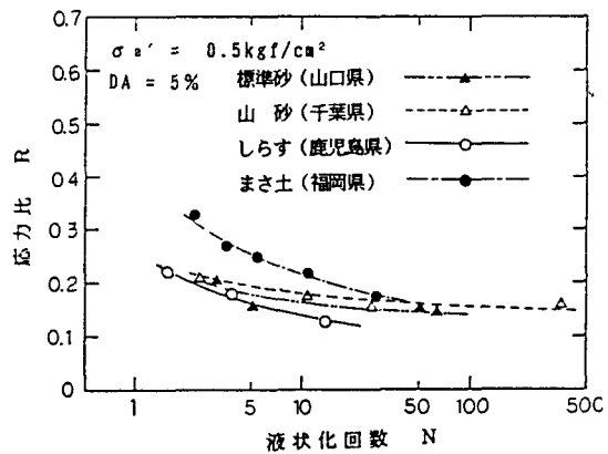
図-4 液状化強度試験結果
