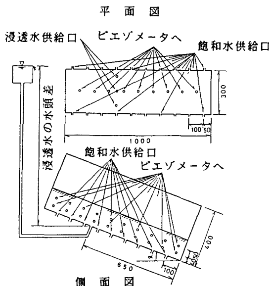
図-1 実験装置の概略図
