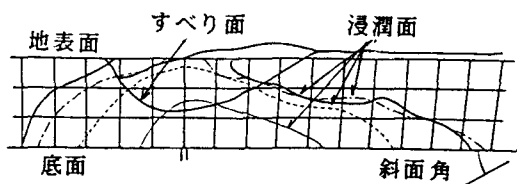
図-5 浸潤面の拡大状況とすべり面
