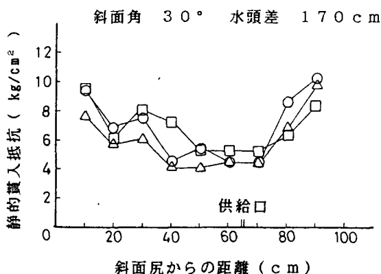
図-4 静的貫入抵抗
