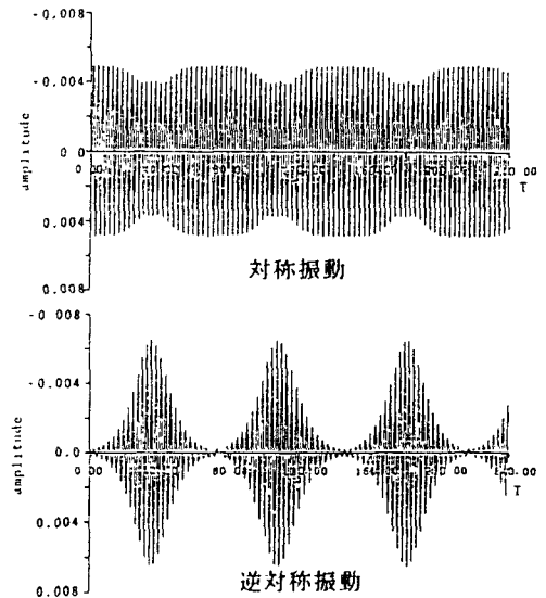
図-5 \gamma=0.10 の副不安定領域における時間応答
