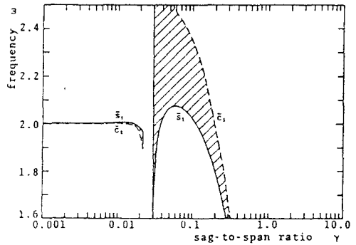
図-4 副不安定領域
