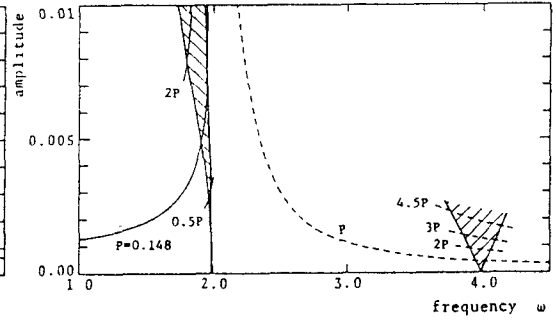
図-3 \gamma=0.03 の応答曲線
