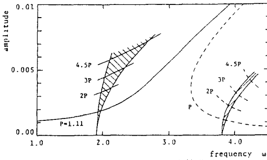
図-2 \gamma=0.10 の応答曲線
