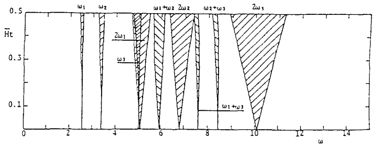
図-3 ケーブルの不安定領域 ( \gamma=0.04, k=30 )
