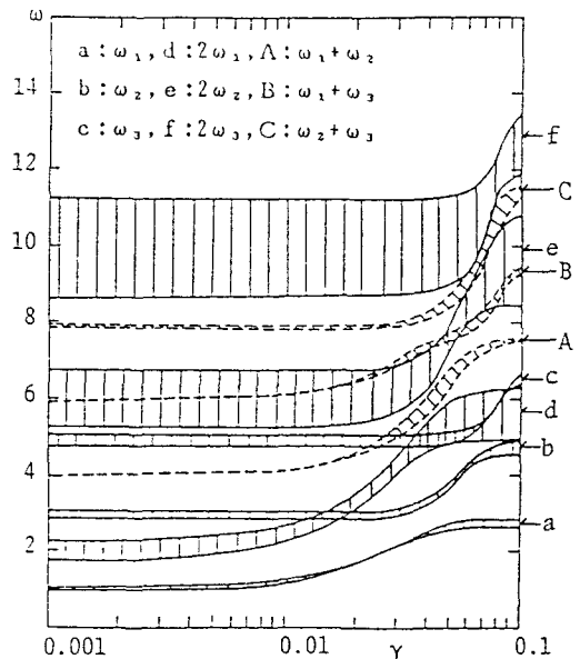
図-4 ケーブルの不安定領域とサグ比の関係
