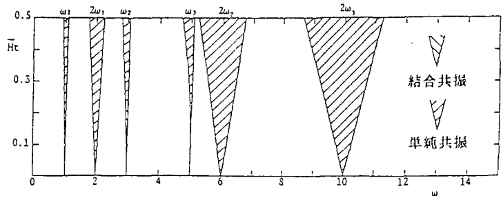
図-2 ケーブルの不安定領域 ( \gamma=0.001, k=30 )
