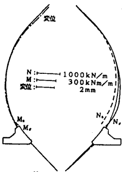
(c) 慣性力の場合 図-6 シェル要素解析
