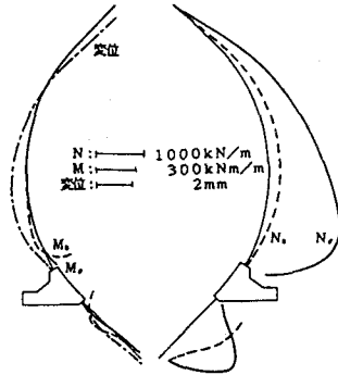
(a) 静水圧の場合 ( \rho = 1.05 \text{ t/m}^3 ) 図-6 シェル要素解析
