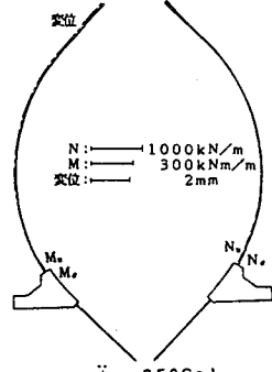
(e) スロッシング圧の場合 図-6 シェル要素解析
