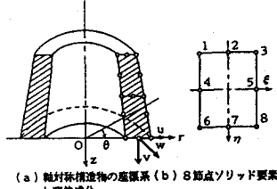
(a) 軸対称構造物の座標系 (b) 8節点ソリッド要素と変位成分 図-3 ソリッド要素解析
