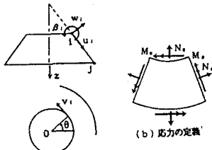
(a) 要素座標系と変位成分 図-2 シェル要素解析
