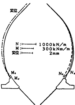
(b) 自重の場合 ( \rho = 2.5 \text{ t/m}^3 ) 図-6 シェル要素解析
