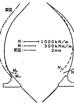
(d) 衝撃圧の場合 図-6 シェル要素解析
