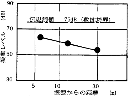
図4 振動測定結果
