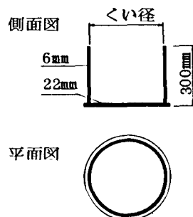
図2 キャップ (先端支持器)
