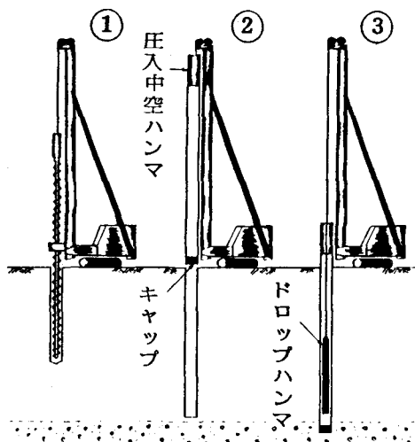
図1 施工方法
