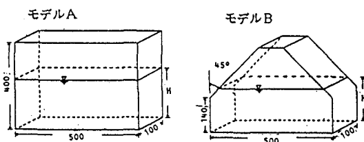
図-1 貯槽模型 (単位mm)
