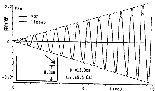
(c) 動水圧の時刻歴応答 (モデルA)
