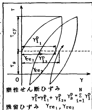
図-4 応力-ひずみ関係
