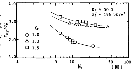
図-3 N_1 と \tau_{cy} / \sigma'_m の関係
