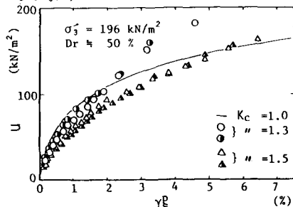
図-5 \sigma'_s と u の関係
