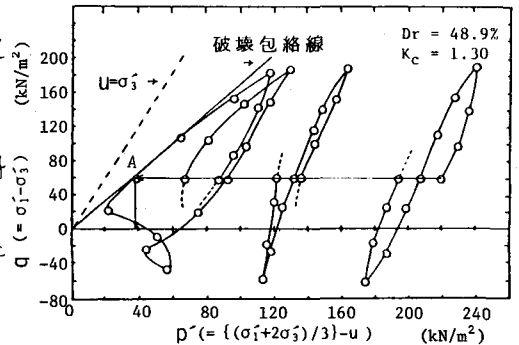
図-1 有効応力径路
