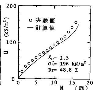
図-8 N と u の関係
