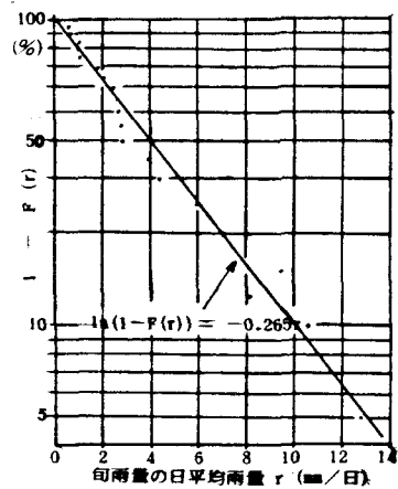
図-1 指数分布の適合性
