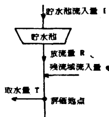
図-4 貯水池モデル
