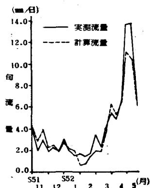
図-3 実測流量と計算流量の比較
