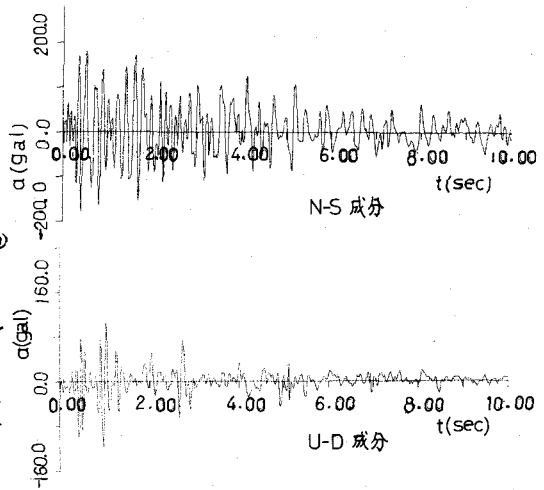
図-1 入力地震波形
