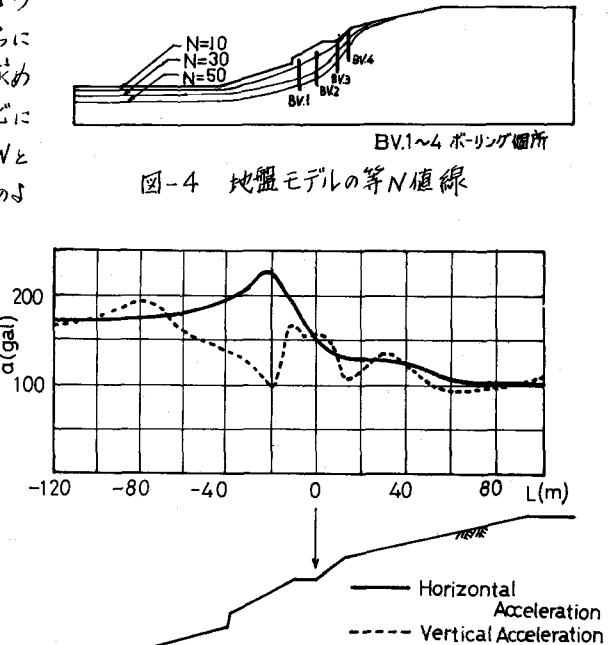
図-5 道路周辺地盤の地表面最大加速度
