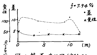
図-6 管の歪と変位図(実験2)
