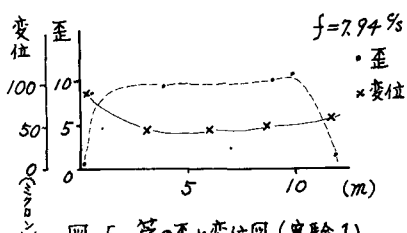
図-5 管の歪と変位図(実験1)
