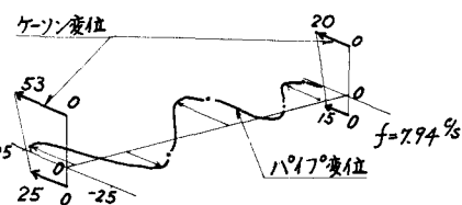
図-7 ケーソンとパイプ(管)変位図
