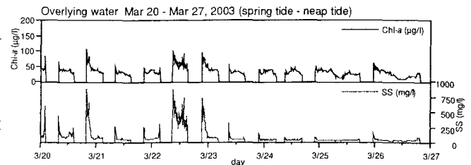
図-3 干潟直上水のChl-aとSS経時変化
