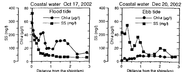
図-4 沿岸水のChl-aとSS岸沖方向分布
