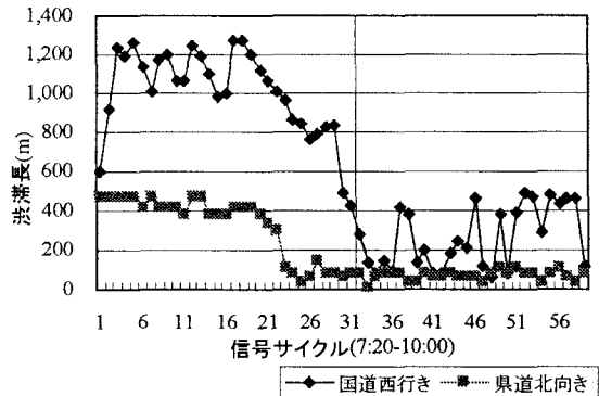
図3 方向別サイクル別渋滞長
