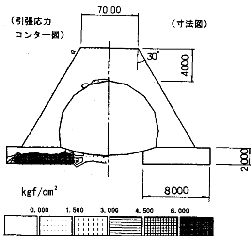
図-3 台形型RCCカルバートに生ずる引張応力コンター図と寸法
