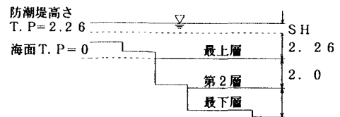
図1 3層メッシュ
