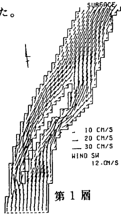
図4 3層メッシュ
