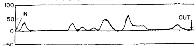
図2 乗船時におけるCase 1の応力波形
