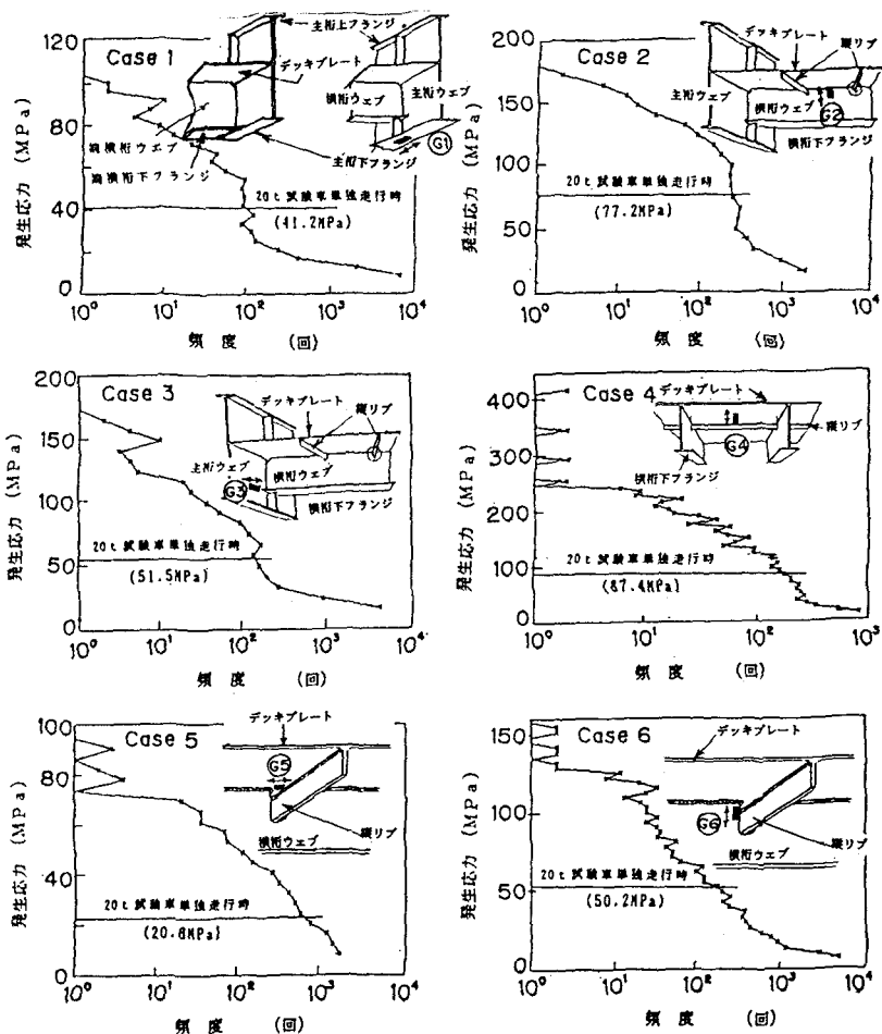
図3 応力 頻度 分布
