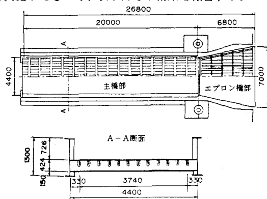
図1 渡橋構造概略図
