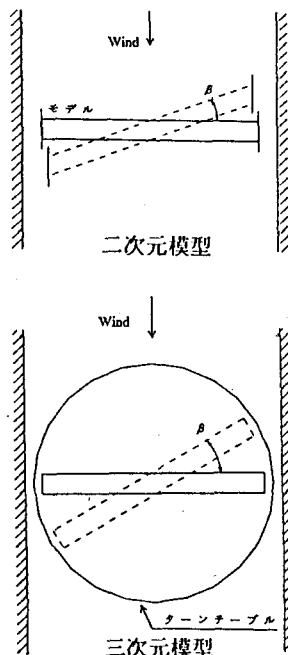
図1 水平偏角 \beta の設定方法 (風洞平面図)
