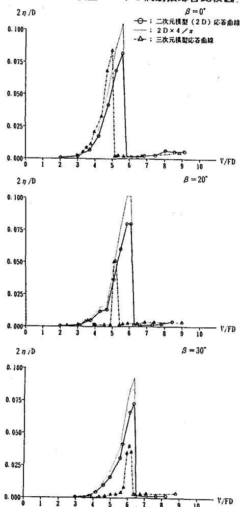
図4 二次元・三次元応答比較図
