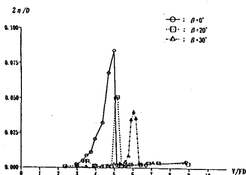
図3 三次元模型における渦励振応答比較図
