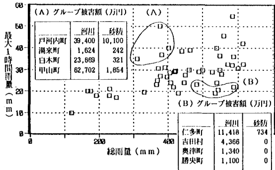
図6 総雨量と最大1時間雨量の関係
