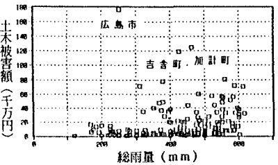
図1 総雨量と土木被害額の関係
