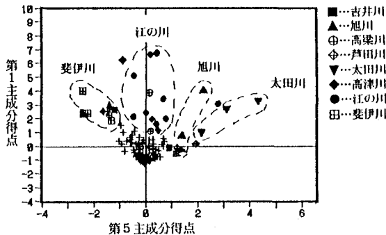
図7 主成分得点の散布図
