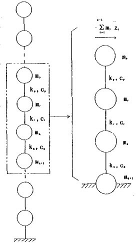
図-1 第J部分系モデル
