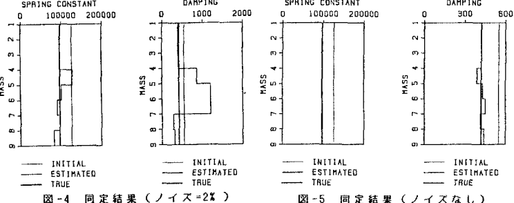
図-4 同定結果(ノイズ=2%)
