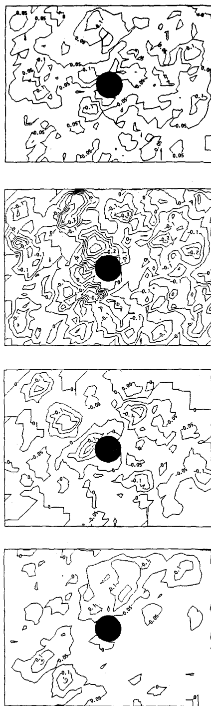
図-3 渦度の等値線
