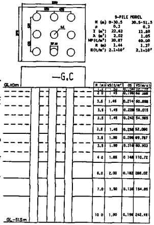
図1 解析対象モデル
