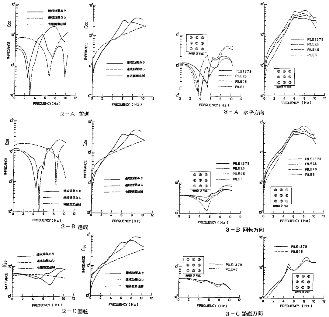
図2 フーチング重心でのインピーダンス
