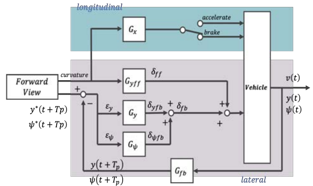
図-1 ドライバモデル
