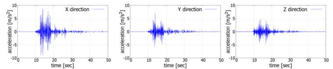
図-3 地震波形(守口観測局 震度5強)
