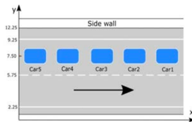
図-4 車両配置
