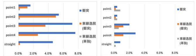
図-8 衝突率(急ブレーキ率 左 20%, 右 40%)
