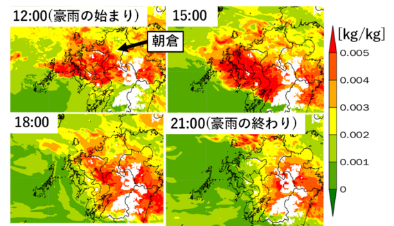
図-6 9 時初期値の予測のばらつきの空間分布図
