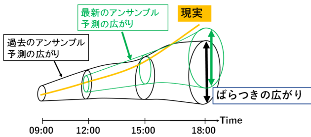
図-3 予測困難な現象に対する特徴(パターン2)
