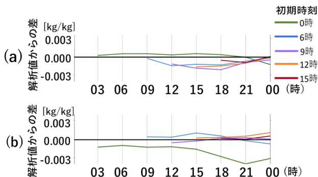
図-4 解析値からの差の推移(正の値は過大予測) (a) 朝倉, (b) 上流側(長崎県の西の海上)
