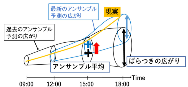
図-1 通常現象に対するアンサンブル予測
