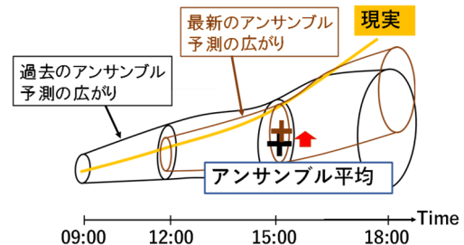
図-2 予測困難な現象に対する特徴（パターン1）
