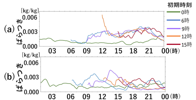
図-5 ばらつき(“アンサンブル最大値-アンサンブル最小値”)の推移 (a) 朝倉, (b) 上流側(長崎県の西の海上)
