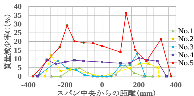
図-3 質量減少率分布
