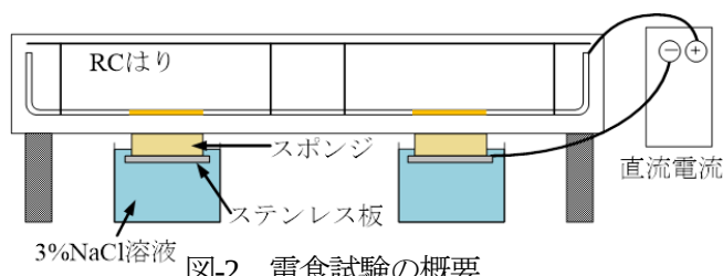
図-2 電食試験の概要
