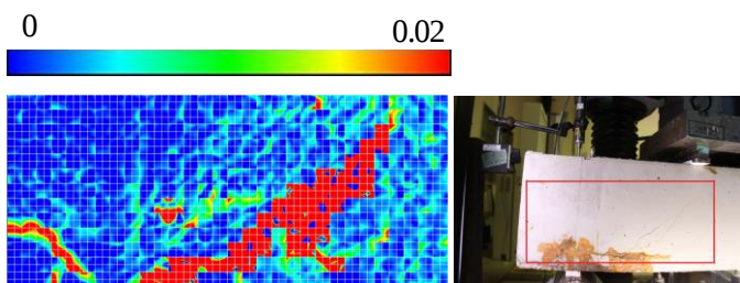
図-5 ピーク後の表面ひずみ分布 (No.2)
