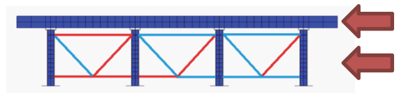
図7 地震時中間対傾構分担メカニズム
