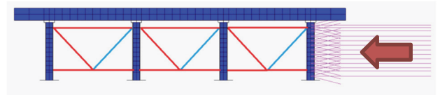
図6 津波時中間対傾構分担メカニズム
