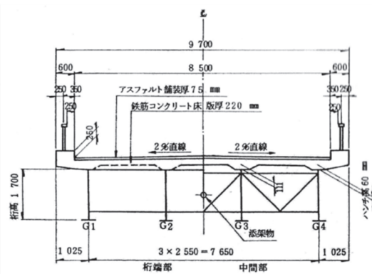
図 1 一般寸法図 2)
