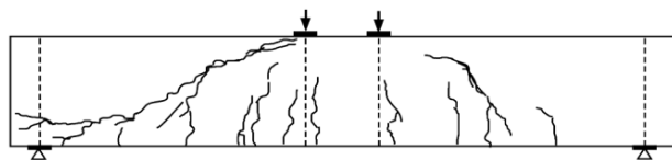
図-3 ひび割れ図 (N-PVA)
