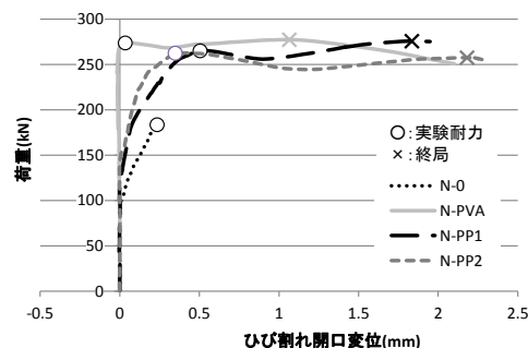
図-5 荷重-ひび割れ開口変位関係
