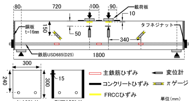
図-2 供試体概要・計測項目
