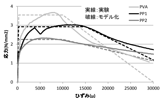
図-1 引張応力-ひずみ関係
