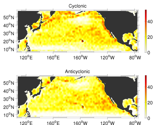
図-2 中規模渦の発生数分布（上：冷水渦，下：暖水渦，2度格子毎の総数）。
