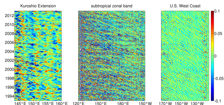
図-4 無次元相対渦度（ \zeta = \nabla \cdot \mathbf{u} / f ）の Hovmöller 図。横軸は経度、縦軸は年。左から、黒潮続流域（38~40°N）、亜熱帯海域（21~23°N）アメリカ西海岸沖（30~32°N）。
