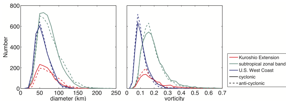
図-3 三海域における渦径（左）および相対無次元渦度（ \zeta = \nabla \cdot \mathbf{u} / f ）（右）ごとの発生数分布。
