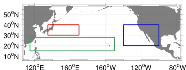
図-1 解析対象領域。赤枠：黒潮続流域，緑枠：亜熱帯海域，青枠：アメリカ西海岸沖。
