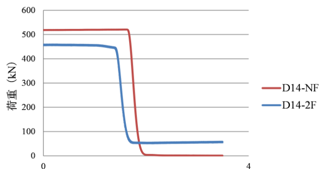
図2 荷重の経時変化
