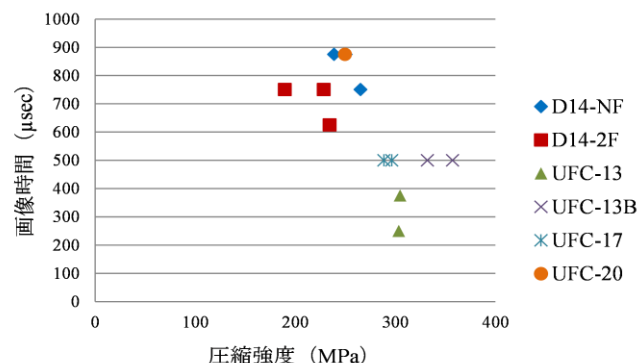
図4 画像時間と圧縮強度
