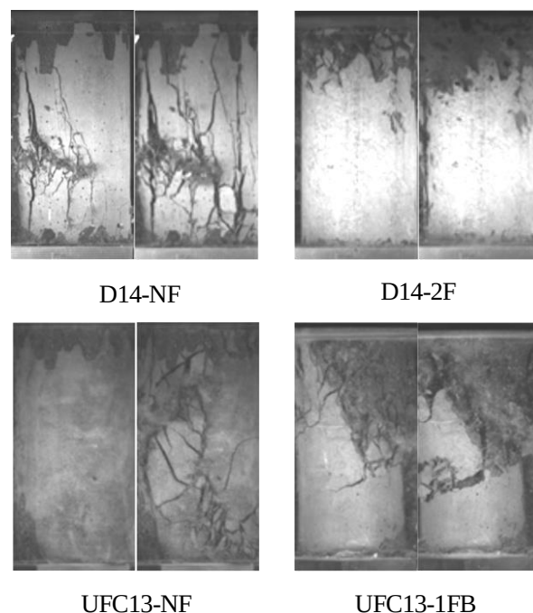
図 1 破壊に至る瞬間の画像
