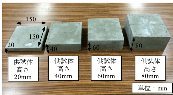
写真-1 モルタル供試体の概要
