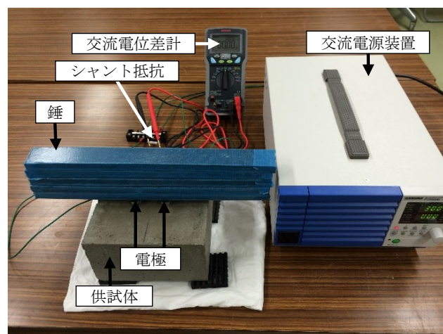
写真-2 二電極法の測定状況
