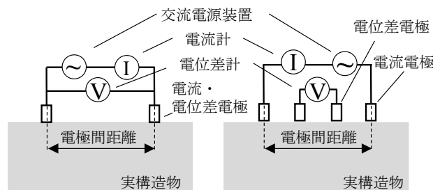
図-1 二電極法
