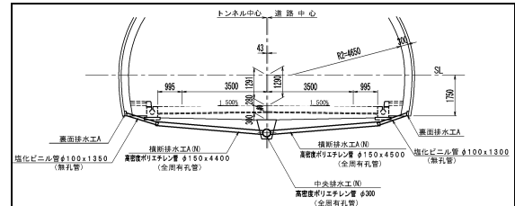
図-1 排水系統概要図
