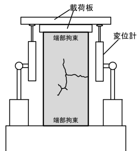
図-1 載荷試験状況
