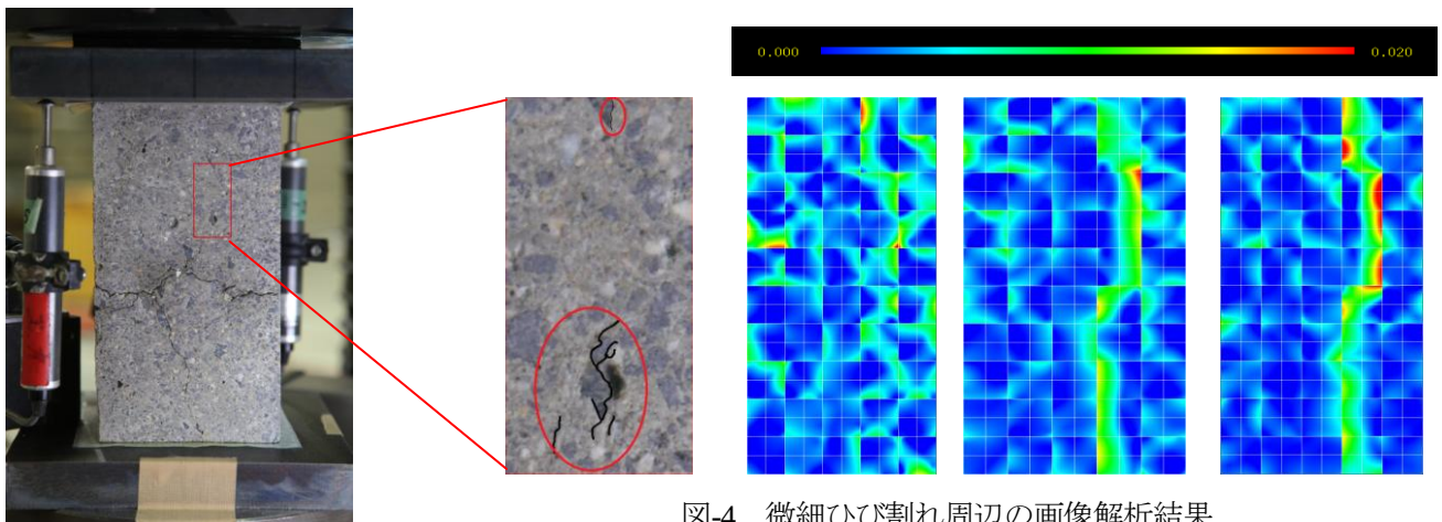
図-4 微細ひび割れ周辺の画像解析結果
